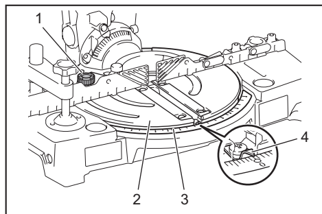
► 1. Vis de fixation 2. Socle rotatif 3. Échelle d'angle de coupe d'onglet 4. Pointeur
