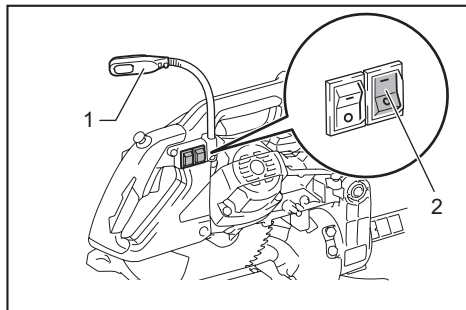
► 1. Lampe 2. Interrupteur de lampe
