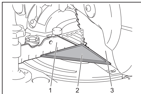
► 1. Garde de guidage 2. Règle triangulaire 3. Lame de scie
