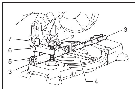
► 1. Bras de l'étau 2. Bouton de l'étau 3. Garde de guidage 4. Socle rotatif 5. Vis inférieure 6. Vis supérieure 7. Tige de l'étau
