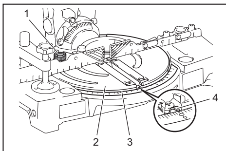
► 1. Vis de fixation 2. Socle rotatif 3. Échelle de coupe d'onglet 4. Pointeur
