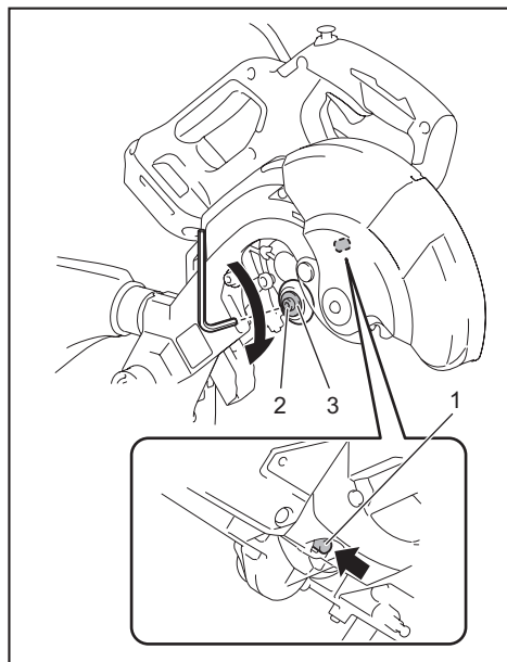
► 1. Blocage de l'arbre 2. Boulon hexagonal 3. Flasque extérieur
