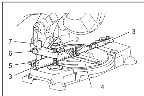
► 1. Brazo de la prensa 2. Seguro de la prensa 3. Guía lateral 4. Base giratoria 5. Tornillo inferior 6. Tornillo superior 7. Varilla de la prensa
