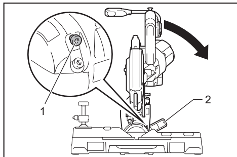
► 1. Boulon de réglage 2. Levier
