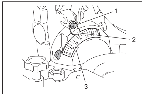
► 1. Vis 2. Pointeur 3. Échelle de coupe en biseau
