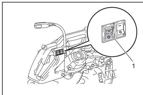
► 1. Interrupteur de laser
