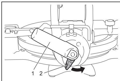
► 1. Levier 2. Levier de libération
